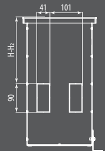
Вид с торца Ntherm Maxi 230 с U-образным бортом
