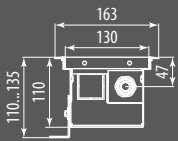
Разрез Ntherm 140.110 с F-образным бортом
