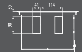
Вид с торца Ntherm 300.200 с F-образным бортом
