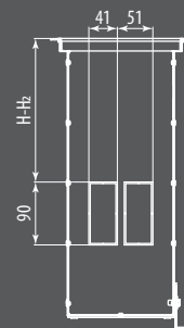
Вид с торца Ntherm Maxi 180 с F-образным бортом
