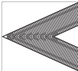
Соединение углом, меньшим 90^\circ с роликовой решеткой
