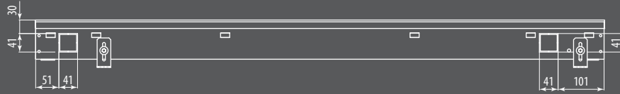
Вид сбоку конвектора Ntherm 140.90 с роликовой решеткой с U-образным бортом
