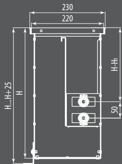
Разрез Ntherm Maxi 230 с U-образным бортом
