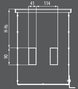
Вид с торца Ntherm Maxi 300 с U-образным бортом
